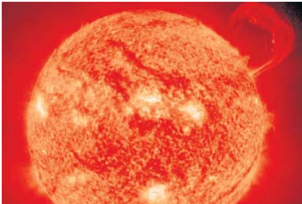
Imagen de una pareja de manchas solares tomada en 2003 por la Torre Solar Sueca.
