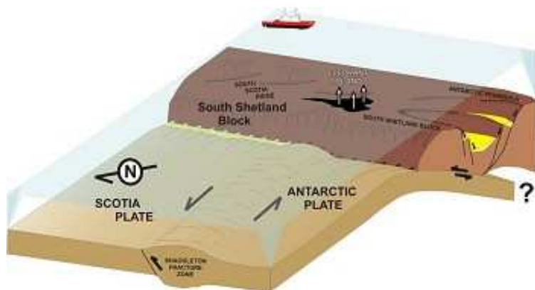
Zona de subducción en el Paso del Drake.
