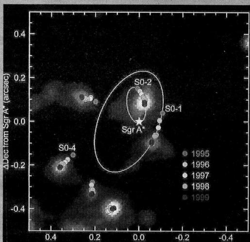
Órbita de la estrella en torno al agujero negro del centro de la Vía Láctea.
