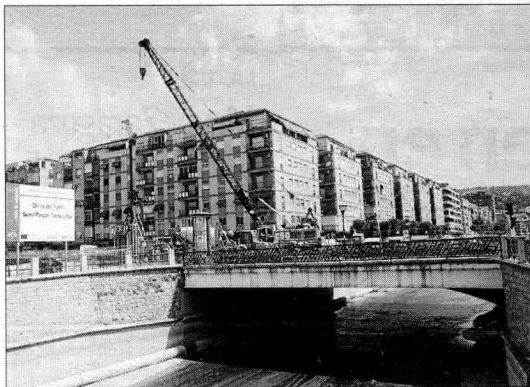
Antes y después. Imagen del puente el pasado día 18 (izq.) y estado en el que se encontraba ayer, con su parte central demolida. JUAN PALMA
