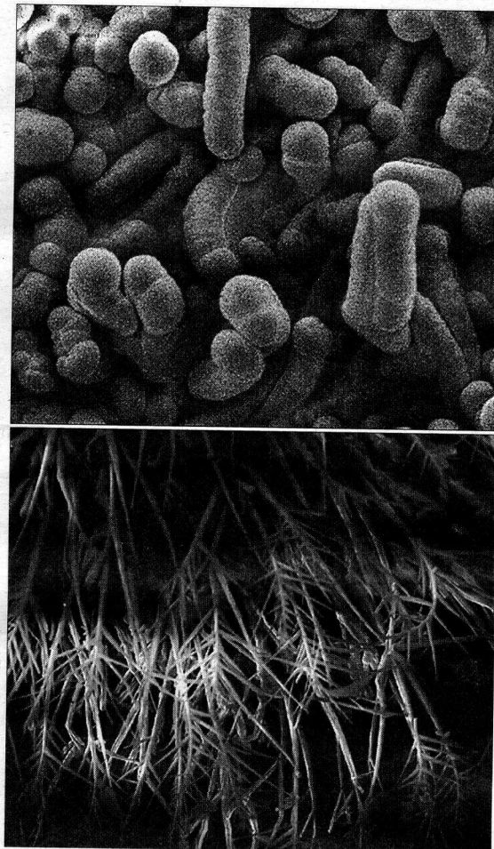
Diminutas estructuras de hielo en forma de palmeras y gusanos. / IACT
